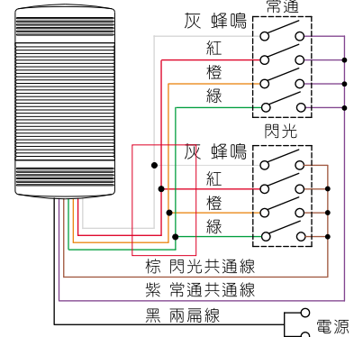
閃光蜂鳴型
